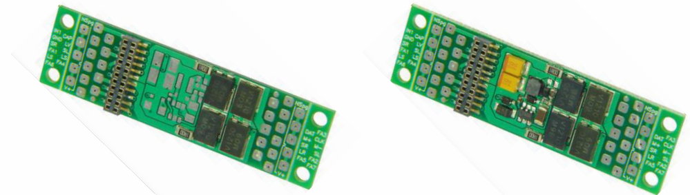
ADAPLU - ohne Niederspannungsquelle ADAPLU15 oder ADAPLU50 - Niederspannung 1,5V bzw. 5V
