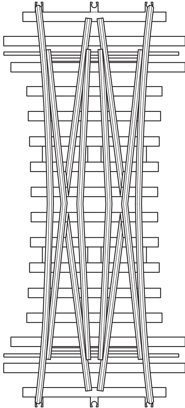
Doppelte Kreuzungsweiche - Mittelteil 59093 (H1101)
